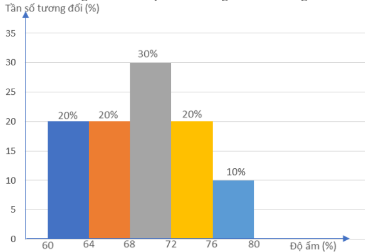
Tần số tương đối của độ ẩm không khí lúc 12 giờ trưa
